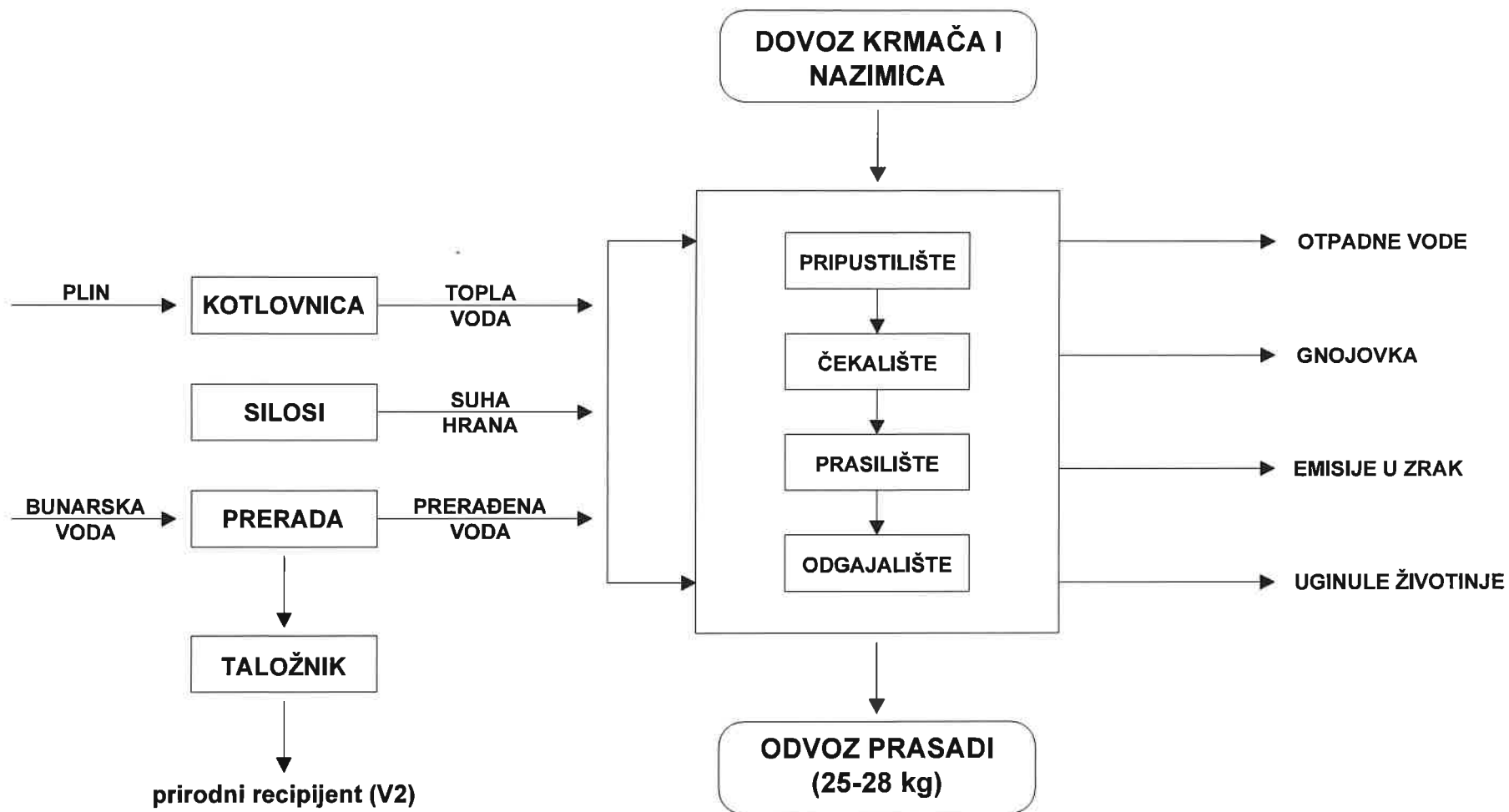
Prilog 2. Blok dijagram tehnološkog procesa na Farmi svinja Haljevo
